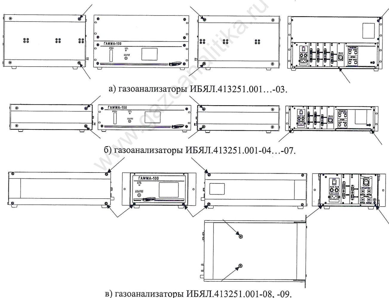
Рисунок 2 - Схема пломбировки от несанкционированного доступа
