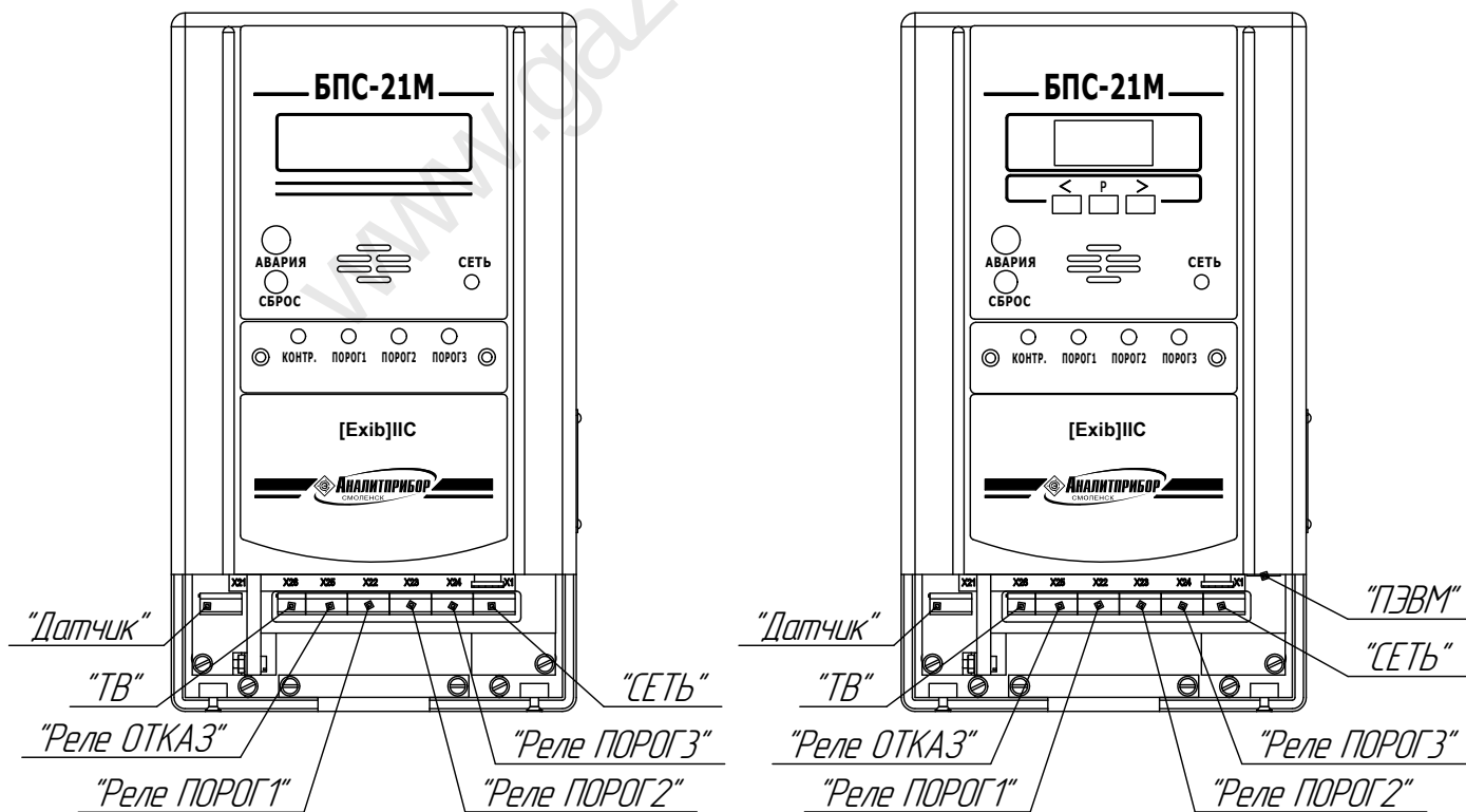
б) блок БПС-21М-1ВБТ
